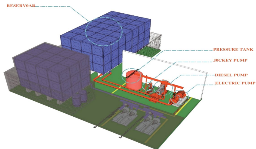
Gambar Sistem Penyediaan Air Kebakaran
